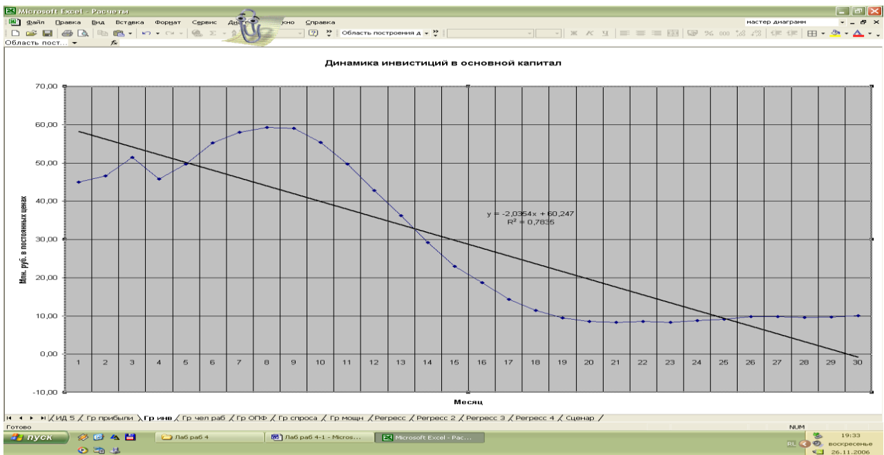
Рис. 3. Графическое изображение линии тренда линейного типа
