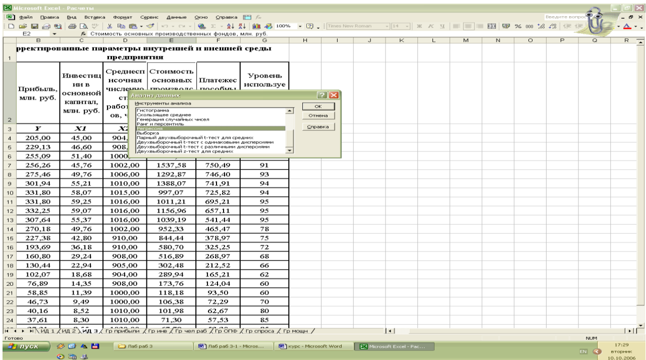
Рис. 4. Выбор режима работы «Регрессия»
