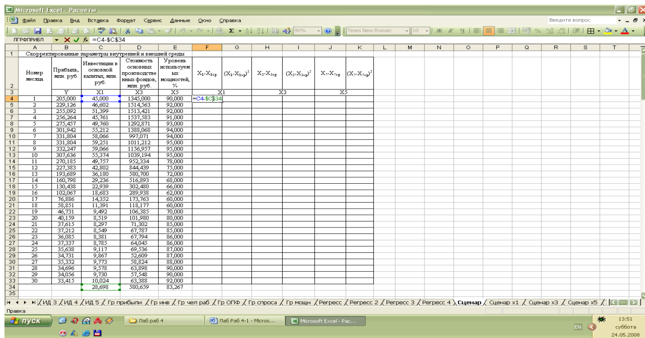
Рис. 21. Нахождение '=X_i - X_{icp}'
